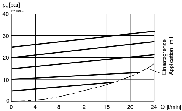
p = f(Q) Druck-Volumenstrom-Kennlinie p_N = 100 bar
