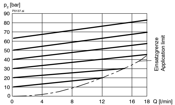
p = f(Q) Druck-Volumenstrom-Kennlinie p_N = 160 bar
