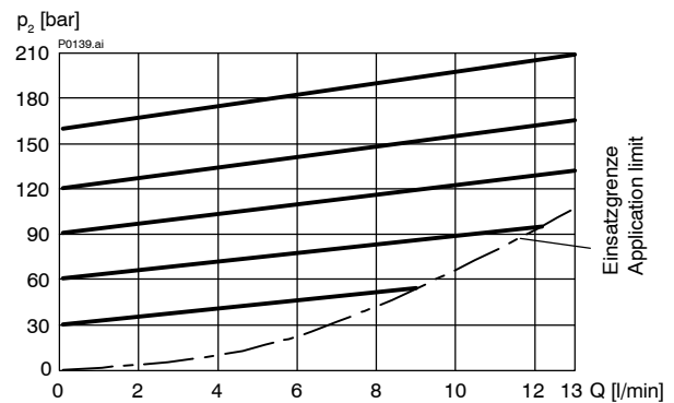
p = f(Q) Druck-Volumenstrom-Kennlinie p_N = 350 bar
