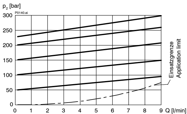
p = f(Q) Druck-Volumenstrom-Kennlinie p_N = 230 bar
