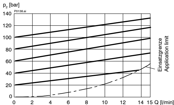
p = f(Q) Druck-Volumenstrom-Kennlinie p_N = 230 bar
