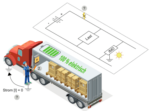
Isolationsfehler in Nutzfahrzeugen werden durch „Insulation Monitoring Devices“ (IMDs) zuverlässig erkannt. Diese Komponente sorgt für eine erhöhte Sicherheit in Elektrofahrzeugen.
