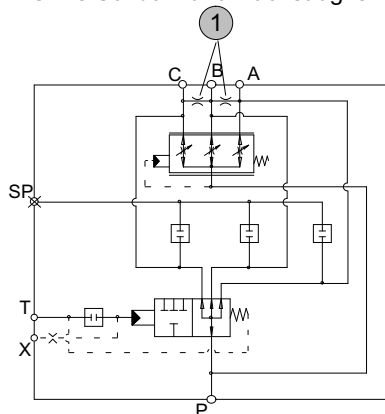
Ohne Schock- und Nachsaugventil
