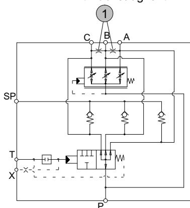
Mit Nachsaugventil
