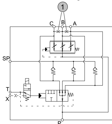
Mit Nachsaugventil
