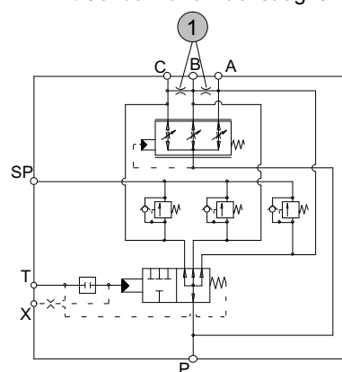
Mit Schock- und Nachsaugventil
