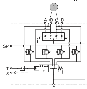
Mit Schock- und Nachsaugventil
