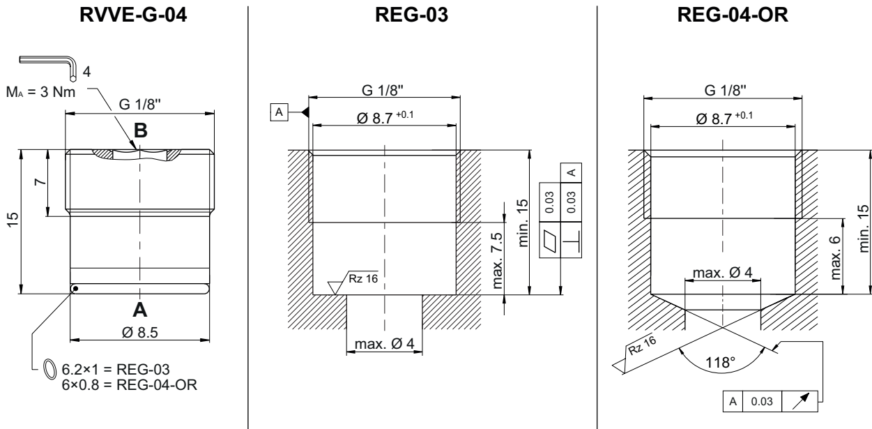
RVVE-G-04 = Rückschlagventil / Einschraubpatrone REG-03 / REG-04 = Abmessung der Bohrungsform für Einschraubpatrone RVVE-G-04
