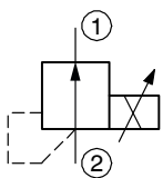
DVSA-1L... DBDRB-1L... DBDSB-1L...
