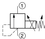
DVSA-1LG DBDRB-1LG... DBDSB-1LG...
